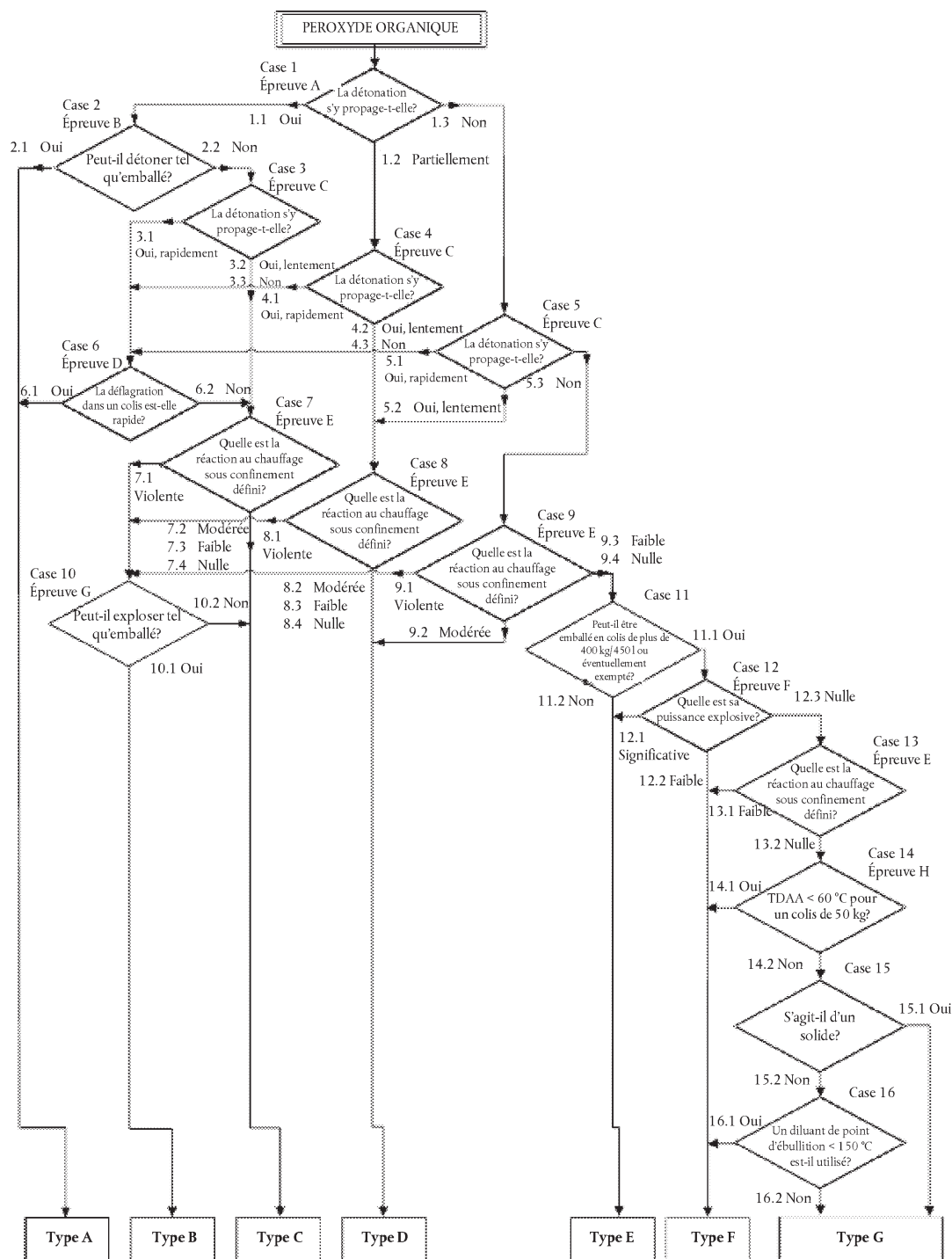
Figure 2.15.1 Peroxydes organiques
